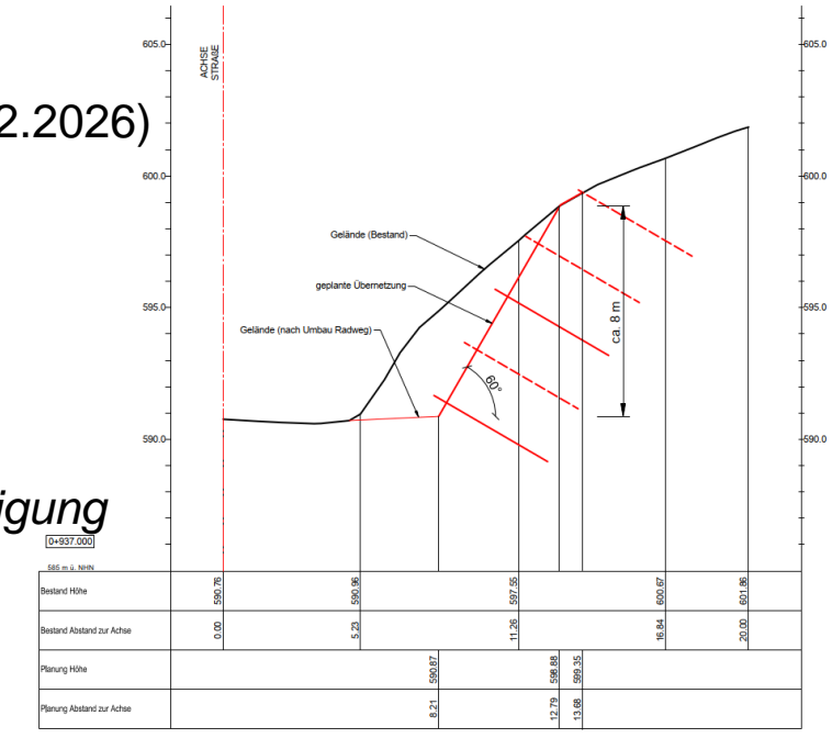
Bsp. Querschnitt Felseingriff
