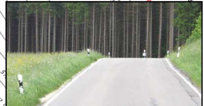
15 Kuppe bei km 2+535, Straße taucht ab, Straßenverlauf nicht erkennbar, Haltesichtweite nicht eingehalten
