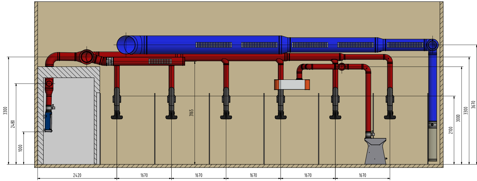
C-C ( 1 : 33 )
